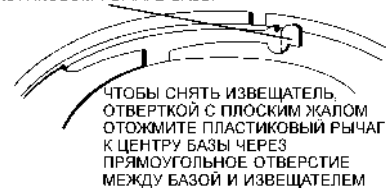
Рис.2. Защита от несанкционированного извлечения извещателя
